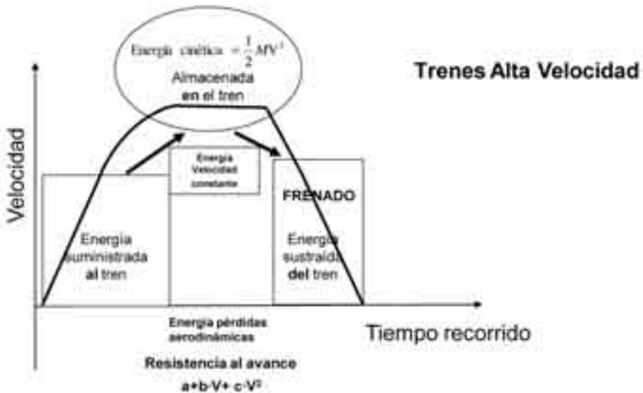
Figura 4 Análisis energético en trenes de alta velocidad
