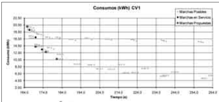
Figura 1 Ejemplo de rediseño en Cuatro Vientos Vía 1
