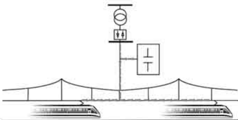
Figura 4 Aprovechamiento del frenado regenerativo
