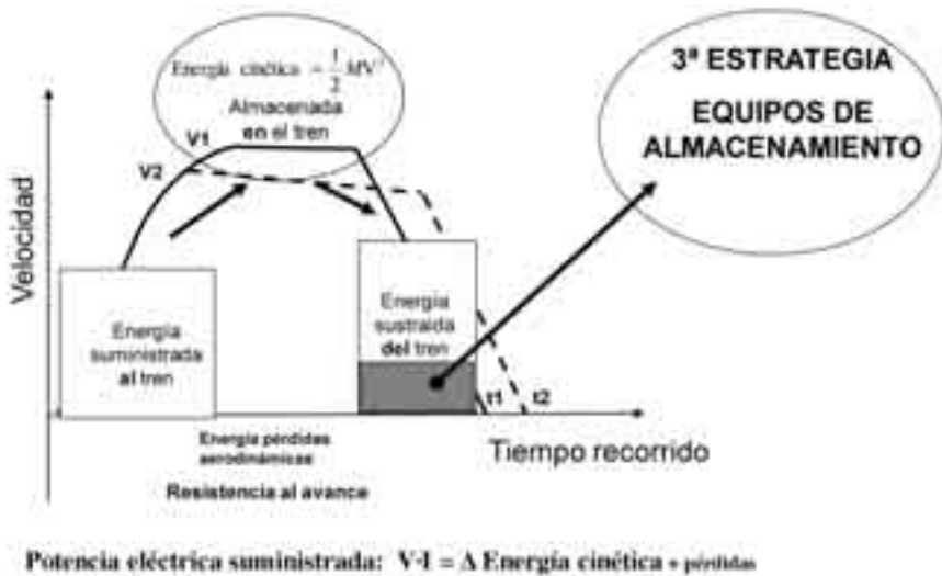
Figura 10 Tercera estrategia de ahorro de energía: Equipos de almacenamiento
