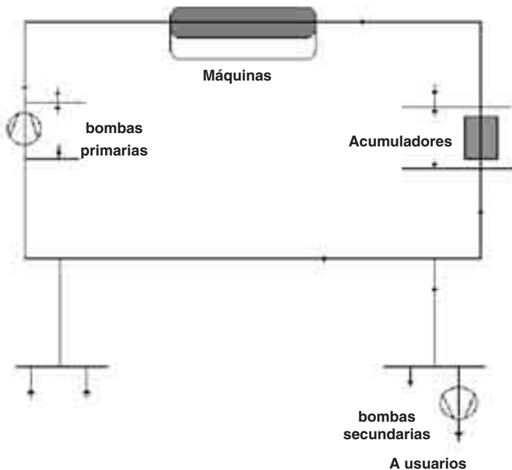
Figura 3 Uso de acumuladores para climatización
