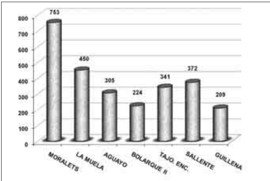
Figura 4 Centrales de bombeo puro en España: Salto neto (metros)
