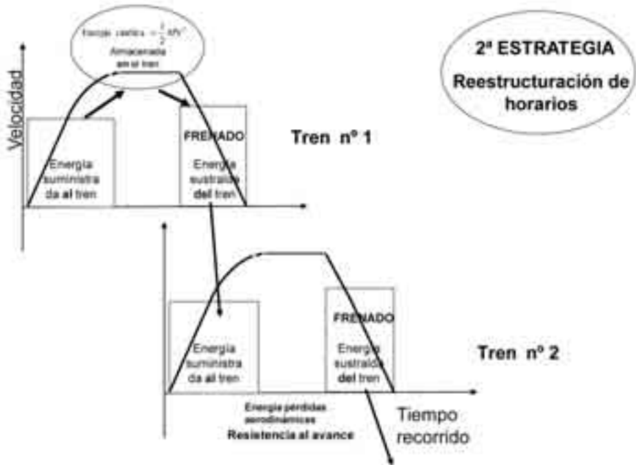
Figura 6 Segunda estrategia de ahorro de energía: Reestructuración de horarios
