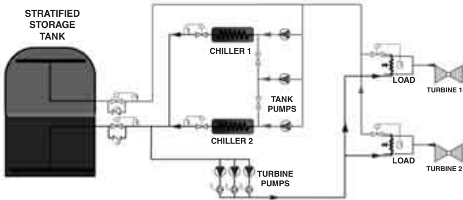
Figura 6 Esquema de principio de la tecnología TESTIAC empleando agua fría estratificada
